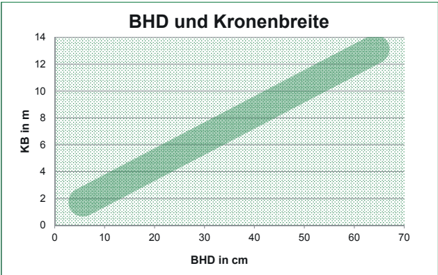
Kronenbreite (KB) in Abhängigkeit vom Brusthöhendurchmesser (BHD) für Laubbäume (Rahmenwerte): Waldbauliche Empfehlungen für die Waldbewirtschaftung in Niederösterreich; 2015; Hochbichler E., Baumgartner L., Schuster K.
